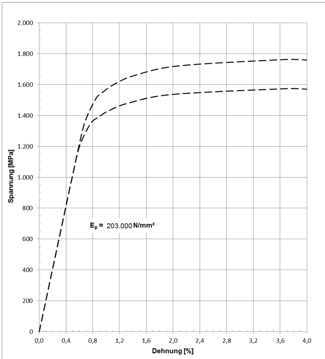
Bild 2: Prinzipieller Spannung-Dehnungs-Verlauf
