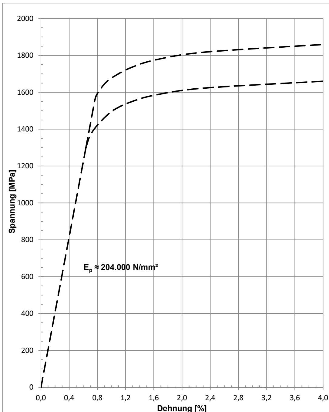
Bild 2: Prinzipieller Spannung-Dehnungs-Verlauf
