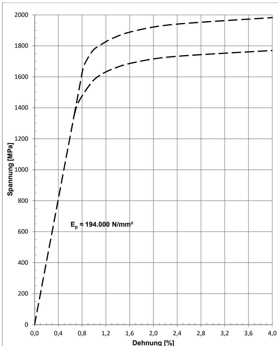
Bild 2: Prinzipieller Spannung-Dehnungs-Verlauf
