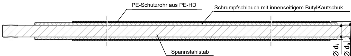
Bild 1: Schematische Darstellung des Zulassungsgegenstandes
