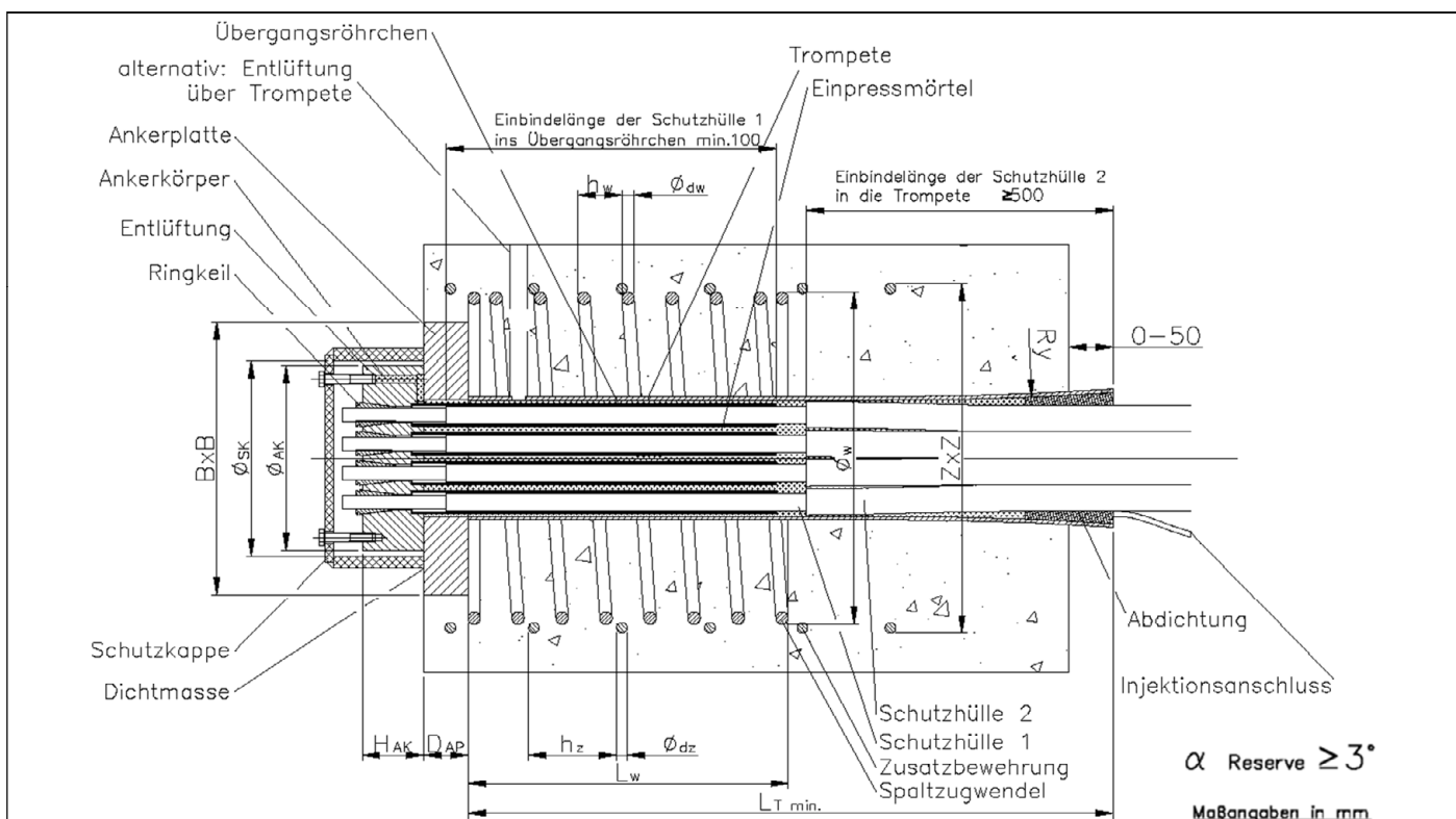
Abmessungen der Verankerungen und Bänder
