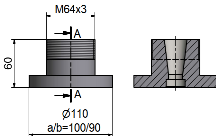
Ankerkopf LoE-1
