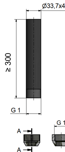
Ankerstützen mit Konusmutter
