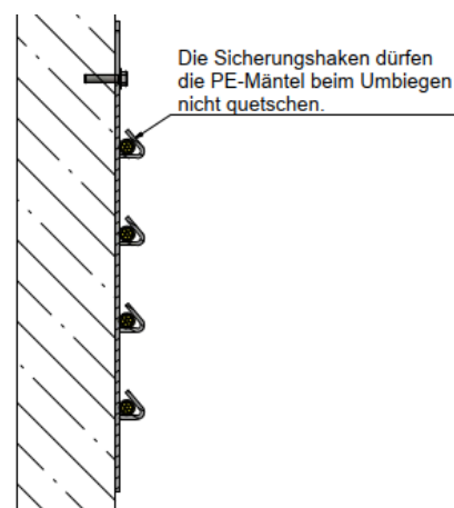
nach der Montage (Schnitt A-A)
