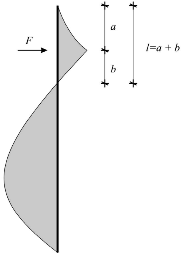
Momentenverlauf
