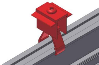
Mittelklemme MH AK II Klick 30-50 ohne Modul
