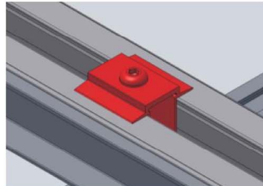
Mittelklemme MH AK II Klick 30-50 mit Modul
