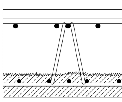
Bild 7: Gitterträger als Verbund- und Querkraftbewehrung (hohe Beanspruchung)
