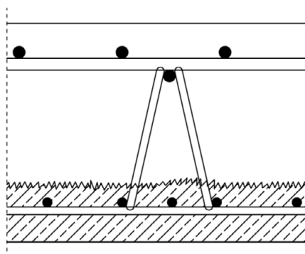
Bild 6: Gitterträger als Verbund- und Querkraftbewehrung (mäßige Beanspruchung)
