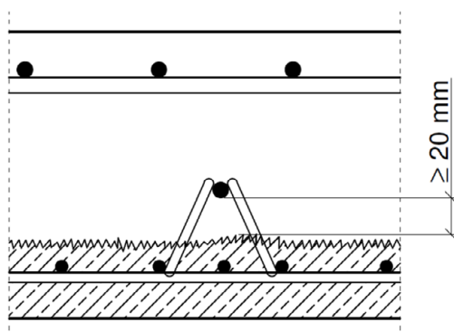
Bild 5: Gitterträger als reine Verbundbewehrung
