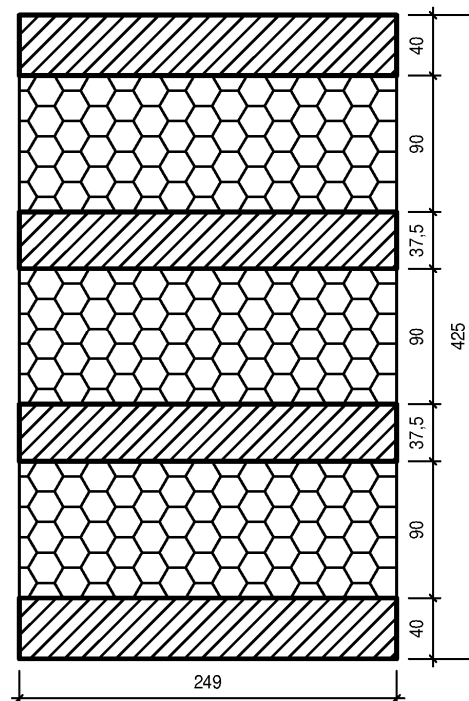
Schnitt B-B
