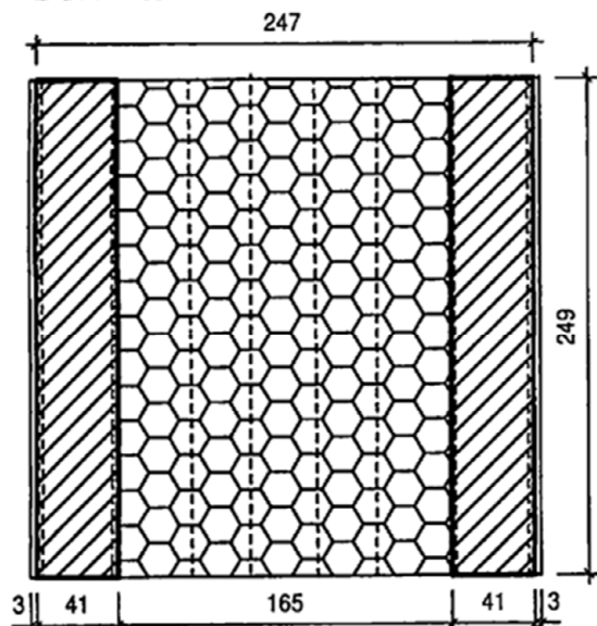
Schnitt A-A
