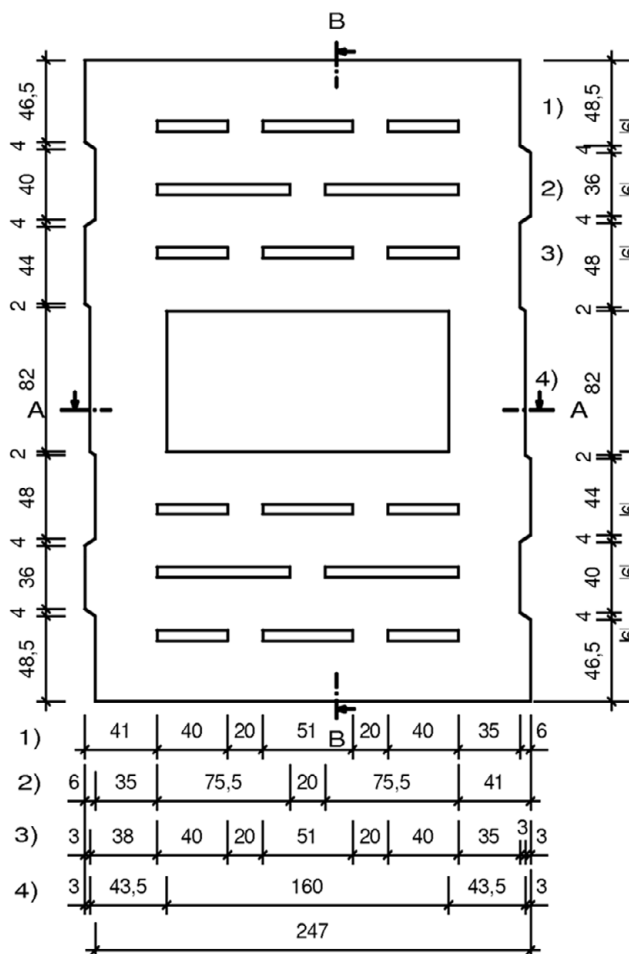
Untersicht
