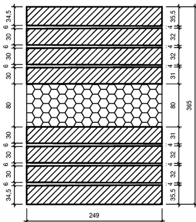
Schnitt B-B
