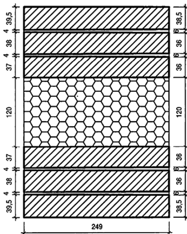
Schnitt B-B
