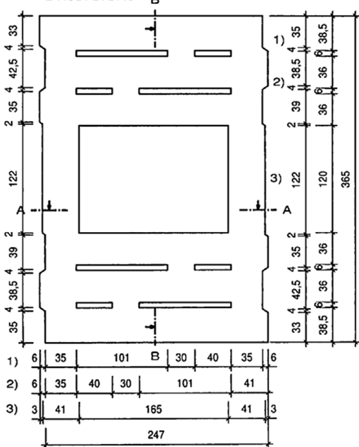
Untersicht
