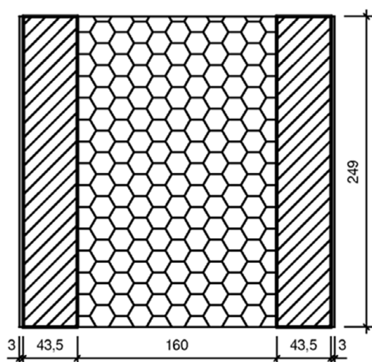
Schnitt A-A
