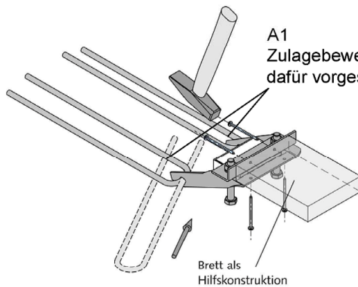
A1 Zulagebewehrung gem. Anlage 12 in dafür vorgesehene Löcher einhängen. A2 Fassadenplattentragteil mit Nägeln an Hilfskonstruktion befestigen (Nagellöcher am Formteil nutzen).
