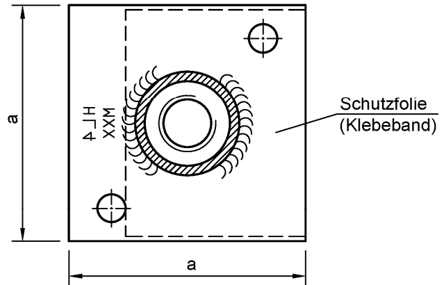
Schnitt A-A
