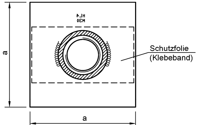
Schnitt A-A
