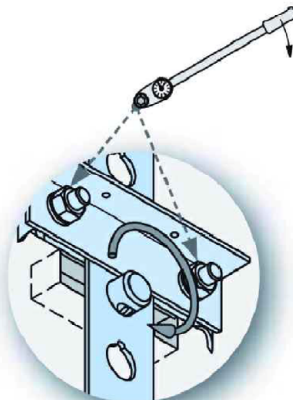
B3 Anzugsdrehmomente für Endmontage gemäß Tabelle 15 auf Mutter aufbringen. Anzugsdrehmomente dürfen nicht überschritten werden.
