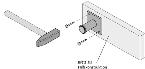
A3 DS3 an Hilfskonstruktion befestigen.
