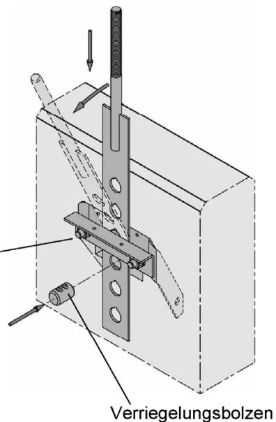
B2 Lochband zwischen Umlenkwinkel und Formteil einführen. Erforderliche Lochbandlänge grob einstellen. Lochband mittels Bolzen verriegeln (Bolzen dabei 180° drehen) und über Umlenkwinkel abbiegen.
