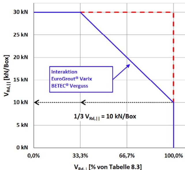
Diagramm 8.1: Interaktion EuroGrout® Varix / BETEC® Verguss
