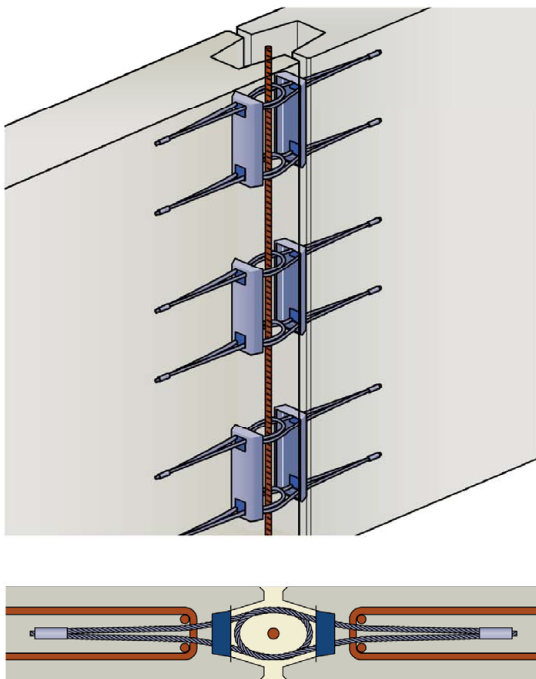
Vertiefter Einbau
