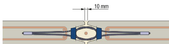
Bild 5.2: Minimale Fuge
