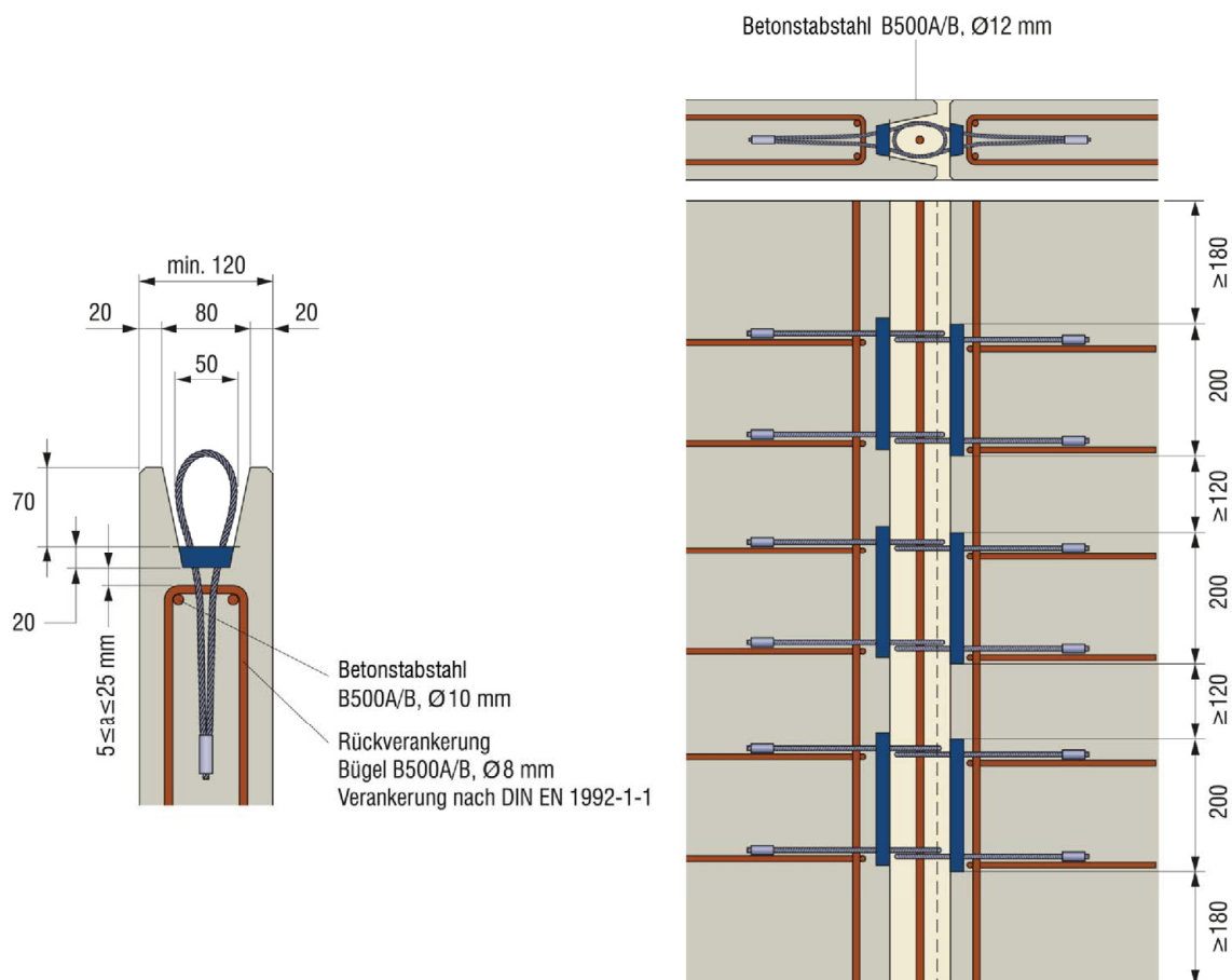
Bild 4.7: Geometrie, Bewehrung (Detail Fertigteil A und B)
