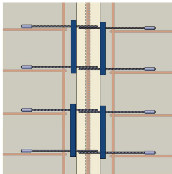
Bild 5.4: Regelfall Schlaufenüberlappung
