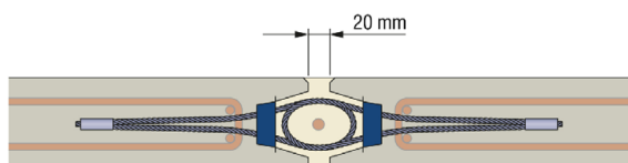
Bild 5.1: Regelfall Fuge
