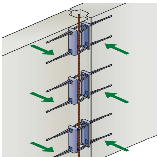
Bild 6.3: Beanspruchung senkrecht zu Fugenlängsrichtung und Wandebene
