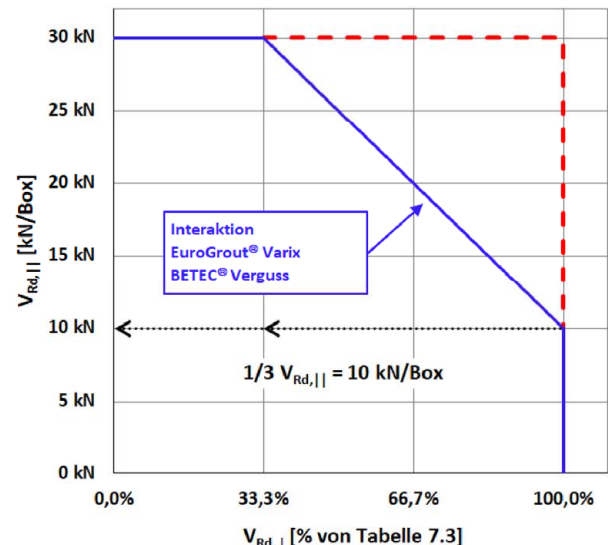
Diagramm 7.2: Interaktion EuroGrout® Varix / BETEC® Verguss
