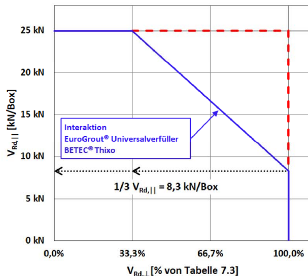
Diagramm 7.1: Interaktion EuroGrout® Universalfüller / BETEC® Thixo
