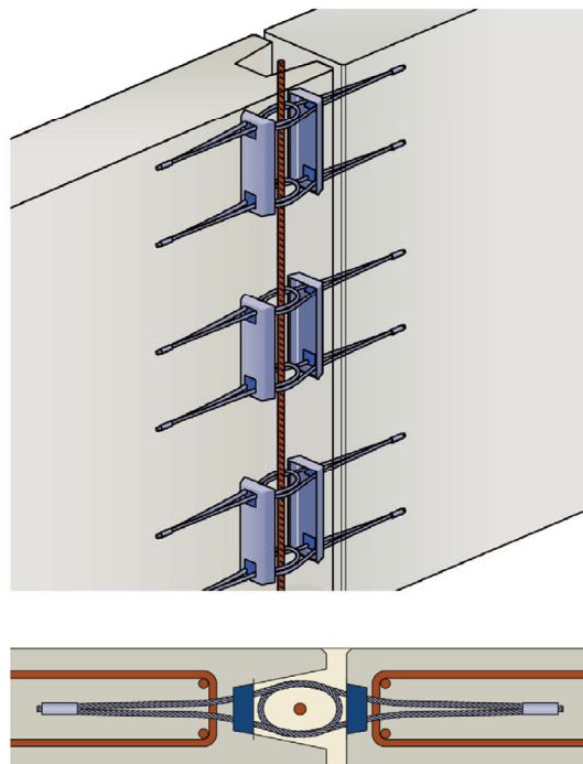
Planer Einbau
