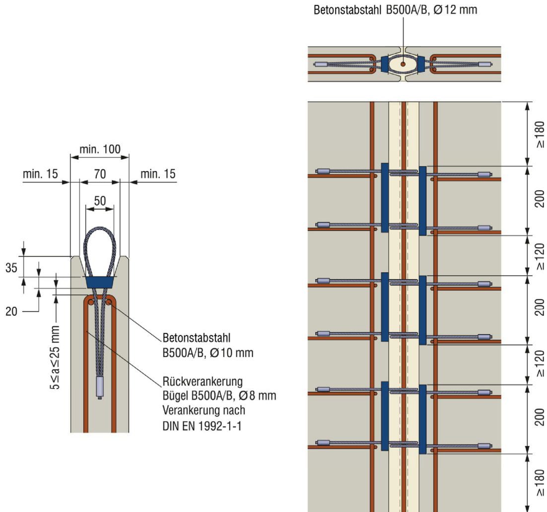
Bild 3.7: Geometrie, Bewehrung (Detail Fertigteil A und B)
