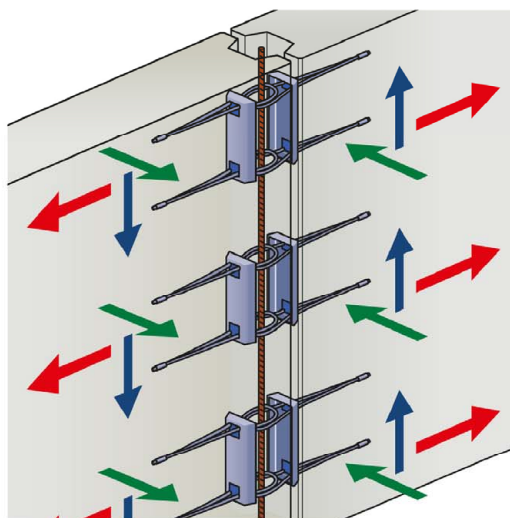
Bild 6.4: Kombinierte Beanspruchung
