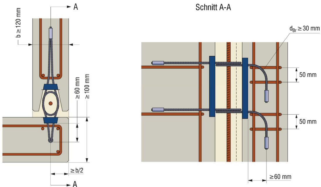
Bild 4.4: Wand – Wand – Eckverbindung - Detail mit abgewinkelten Seilschlaufen
