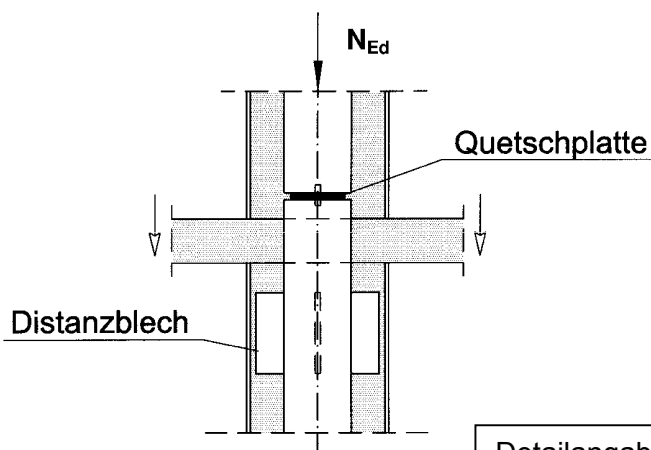
Beispiel für einen Stützenstoß
