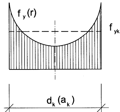
Streckgrenzenverteilung
