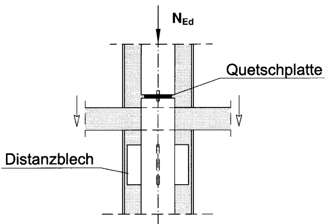
c) Lasteinleitung über das Kernprofil und den Beton
