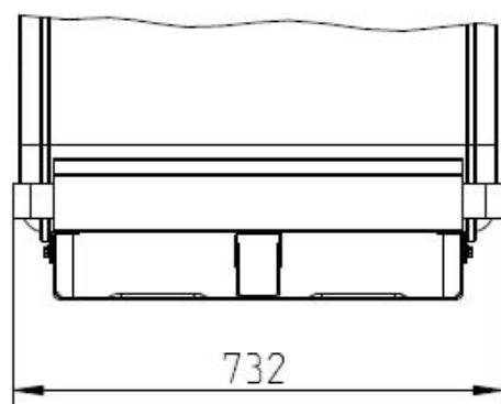
Fußgestell UT 400 mit Anfahrerschutz H = 100 mm; Montageskizze
