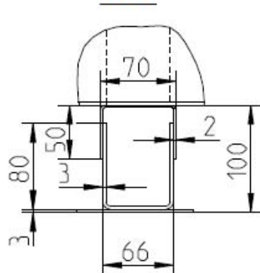
Detail C 0.200
