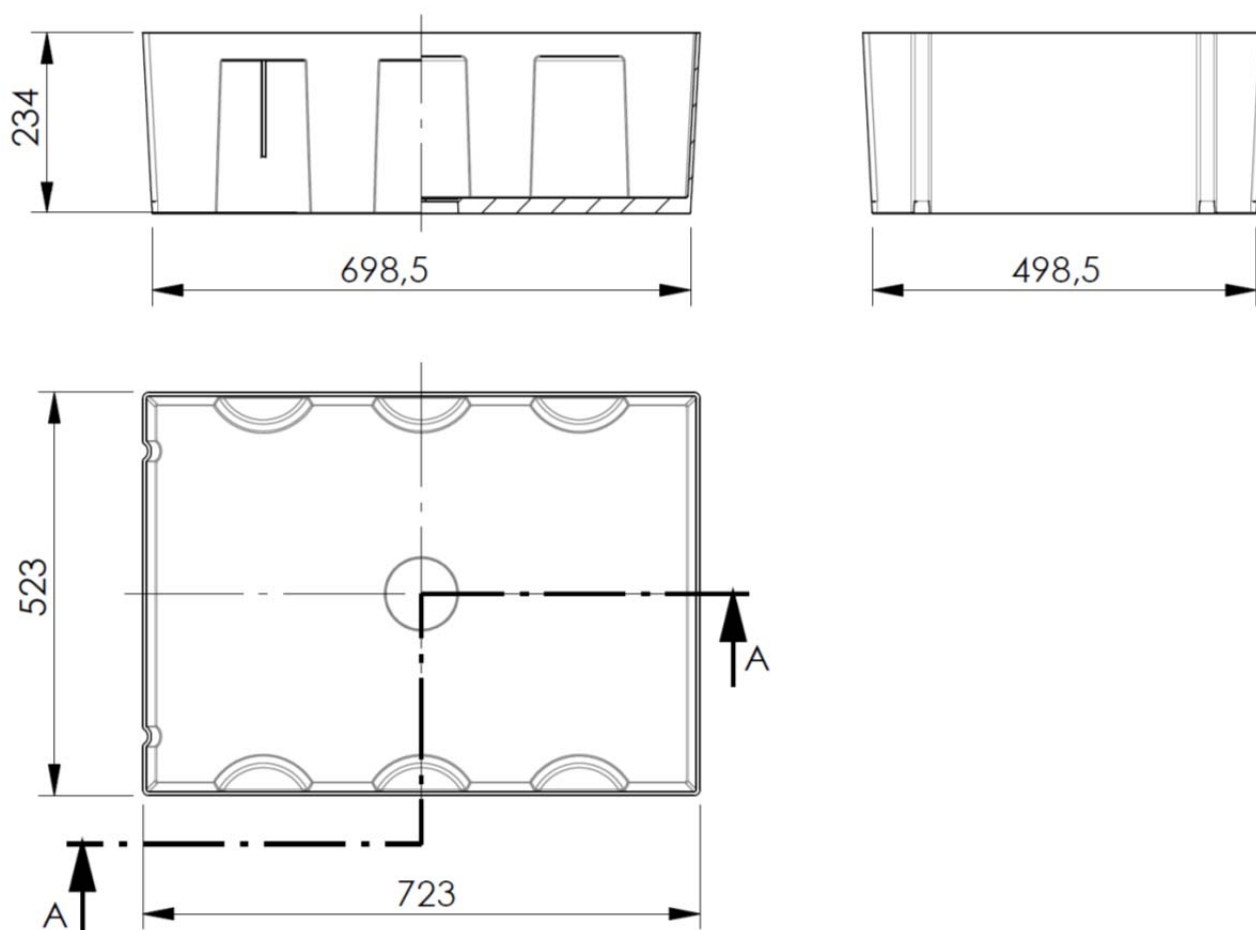
Schnittdarstellung A-A
