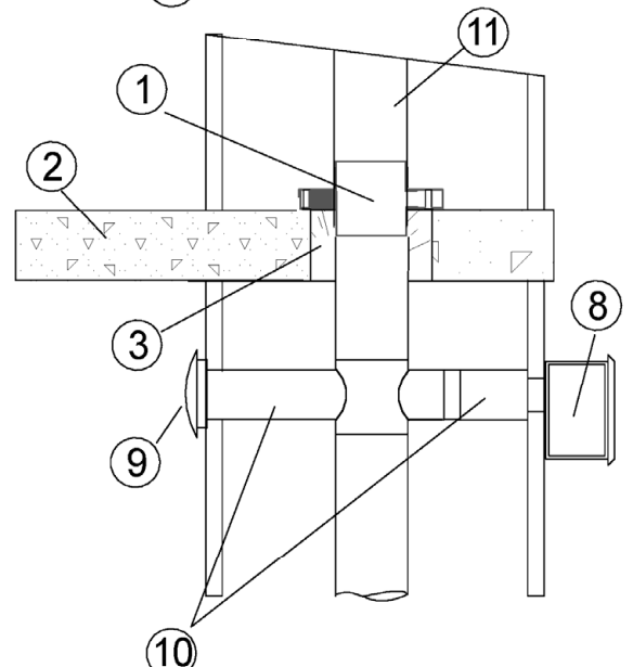
Einbausituation mit Einzellüftungsgeräten
