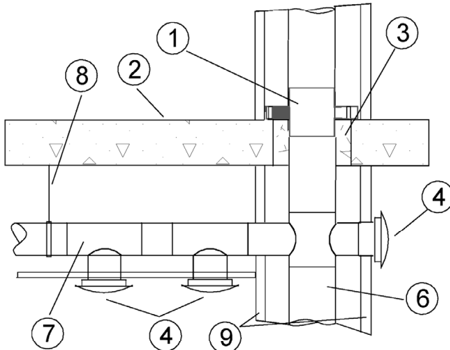
Einbausituation mit Zentrallüftungsanlage
