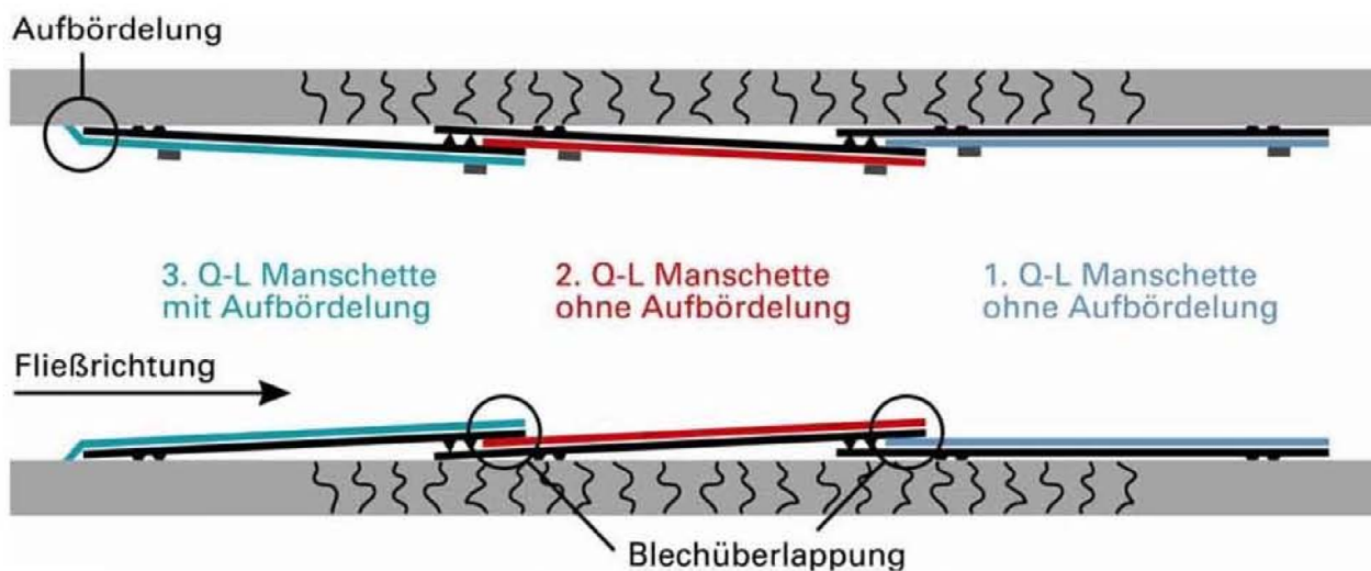
: Serienversetzung Quick-Lock, letzte Manschette gegen Fließrichtung ist aufgebördelt
