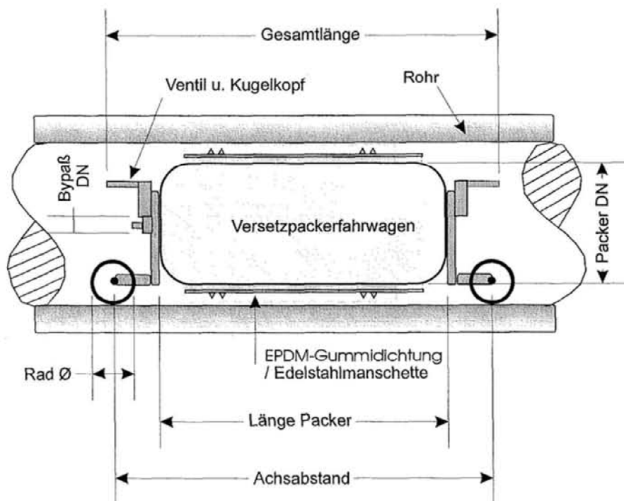
Bild1: Längsschnitt
