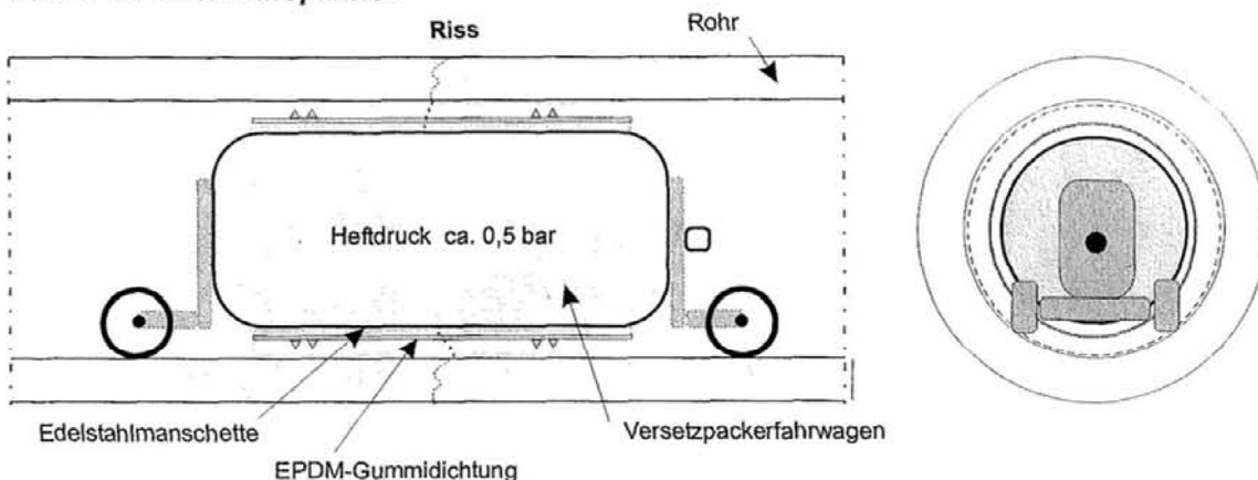
Bild 1: Vor dem Aufspannen
