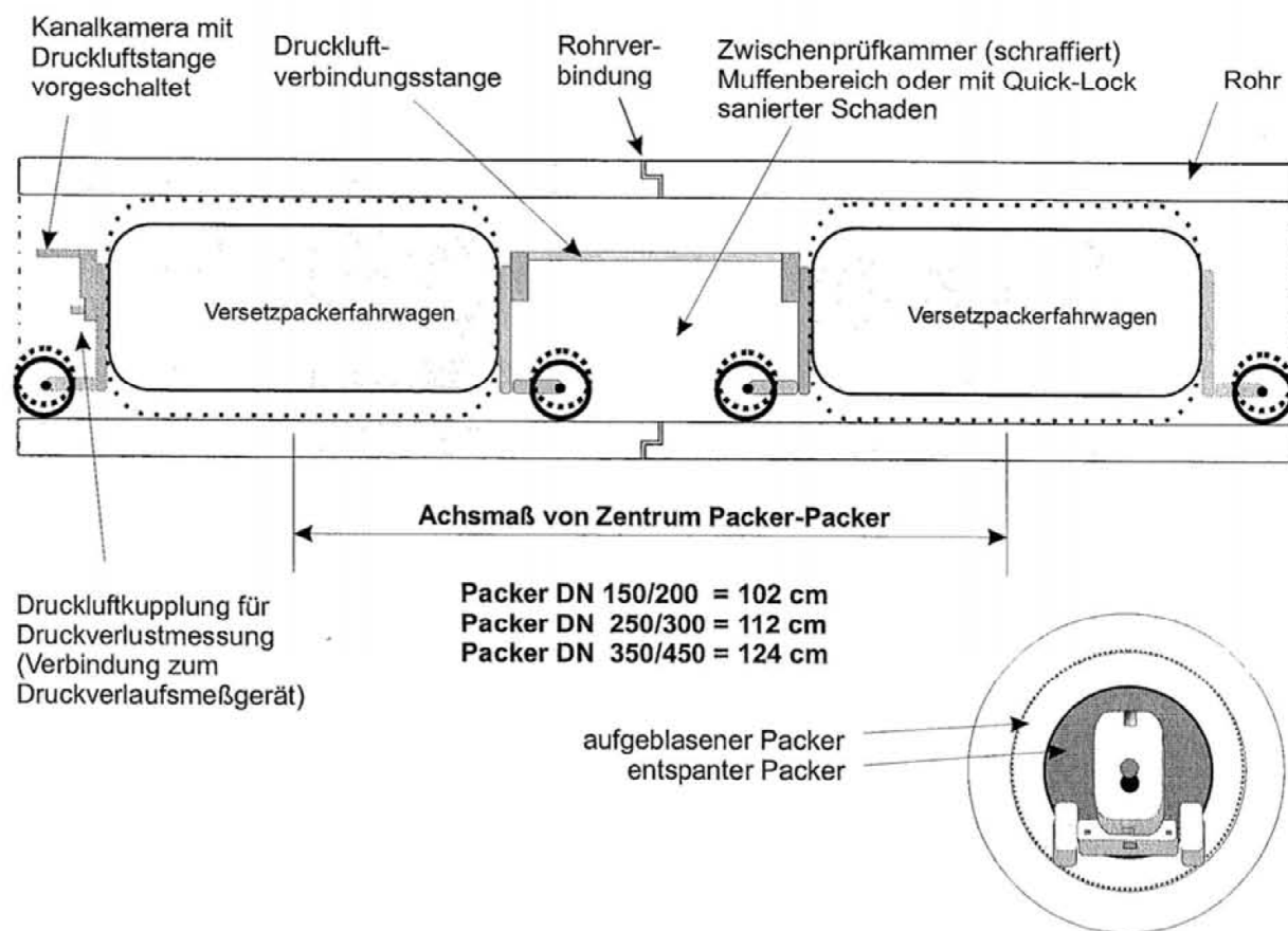
Bild1/2: Längs-/ Querschnitt des Quick-Lock-Tandem bei einer Druckprobe (Packerblasen gefüllt sind gestrichelt dargestellt)
