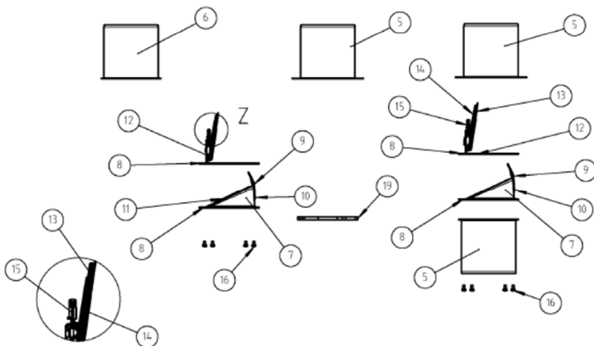
Absperrvorrichtung Silvento-BSK für Brandschutzgehäuse
