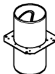
Absperrvorrichtung Silvento-BSK Typ 8/BS für Schachtwandmontage
