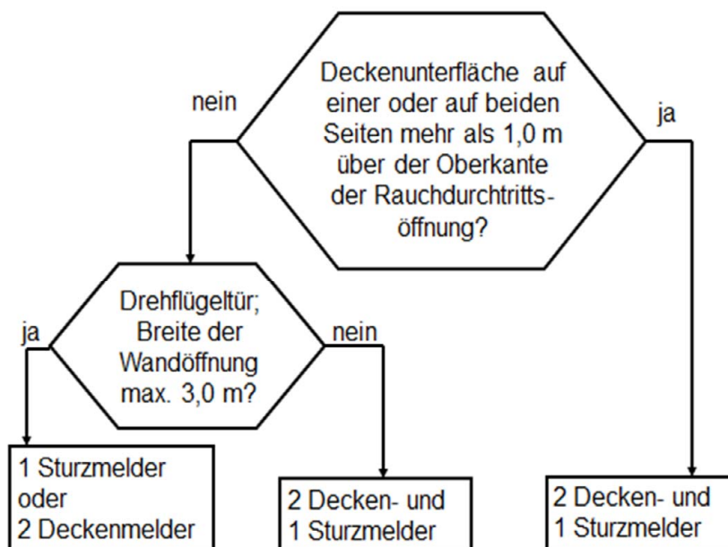
Bild 3: Entscheidungsdiagramm
