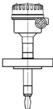
Flanschmontage (mit Verlängerung)
