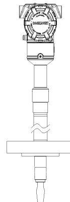
Flaschmontage (mit Standardlänge)
