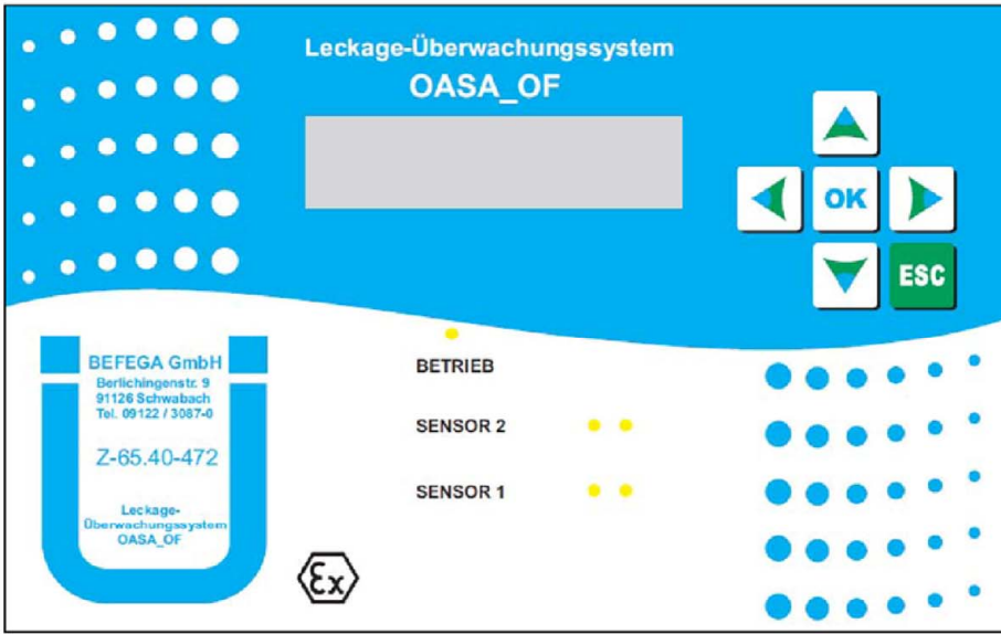
Anzeigegerät OASA_OF
