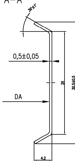
Schnitt A-A
