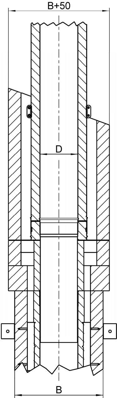
A-A 1:8
