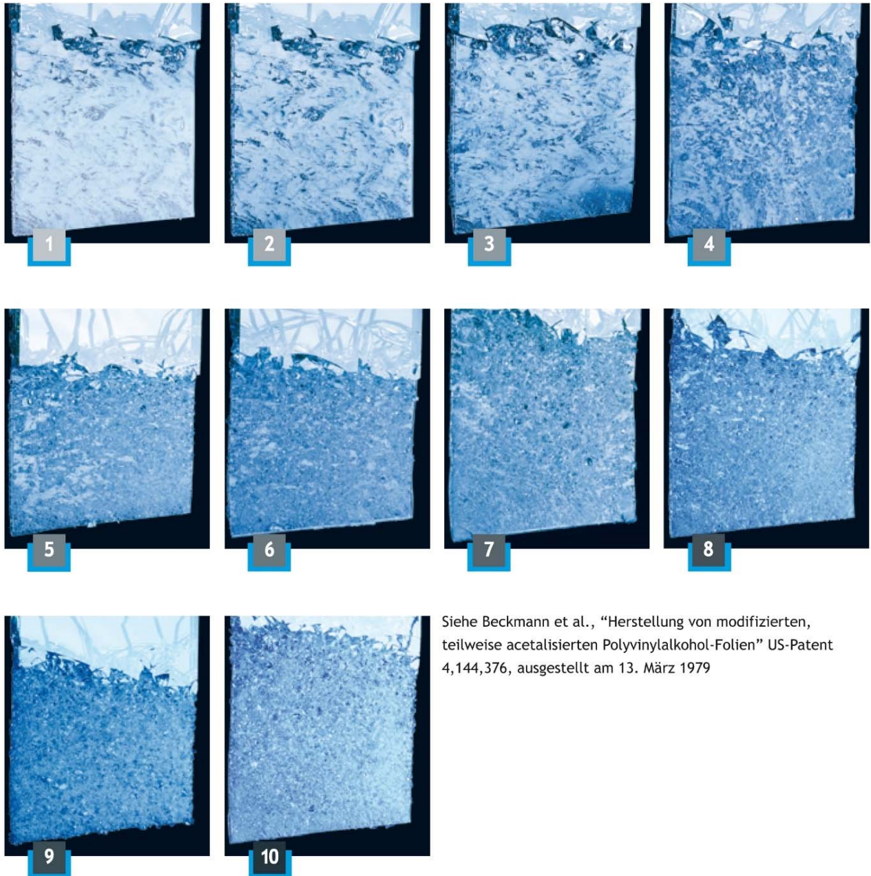
Abb. 3.2: Referenz-Pummelbilder
