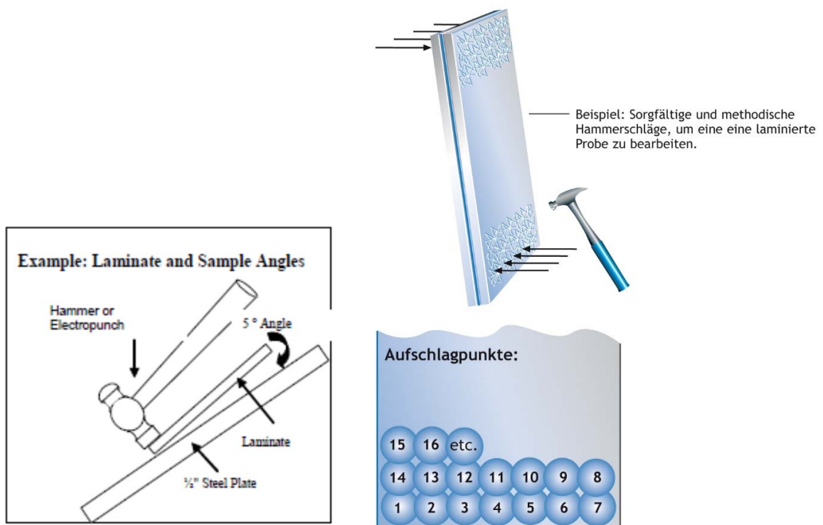
Abb. 3.1: Prüfdurchführung
