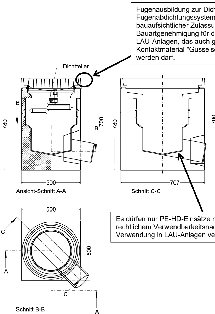
KS2-EK01 - 1: Ablaufelement 1-teilig Pult mit Dichtteller und Gusseisenrost
