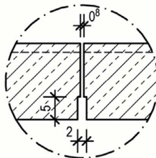
DETAIL VERBINDUNGSFUGE
