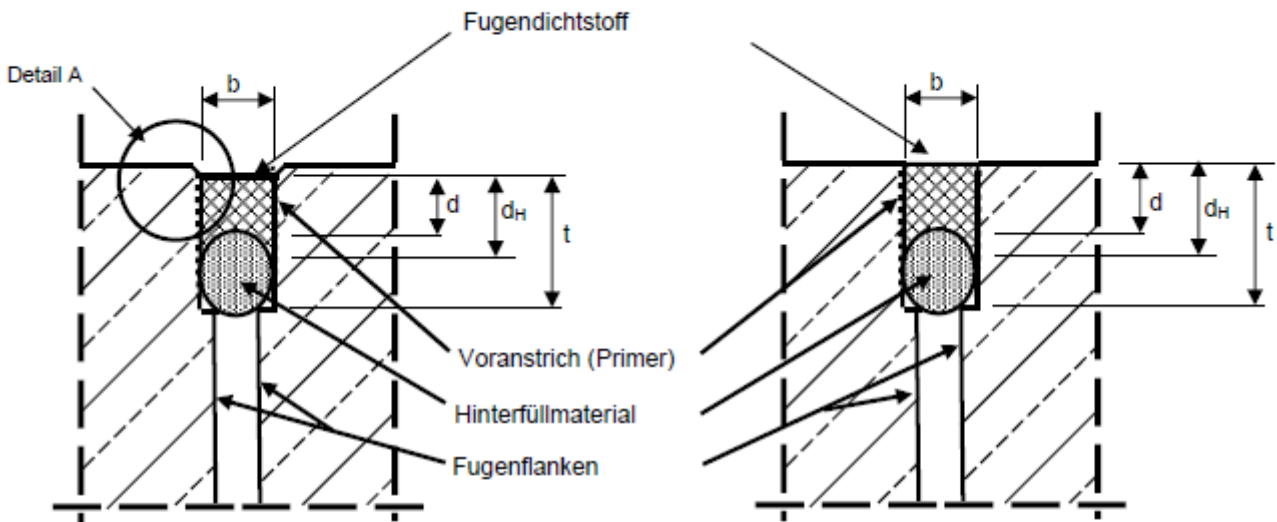
befahrbare Fugenkonstruktion
