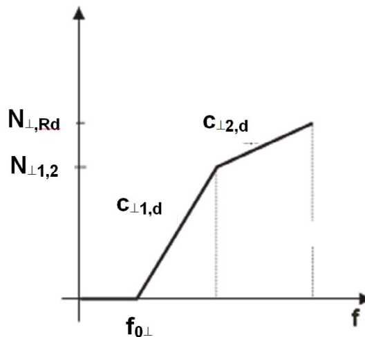
Bild 4: Trilineare Steifigkeit c_{\perp,d}
