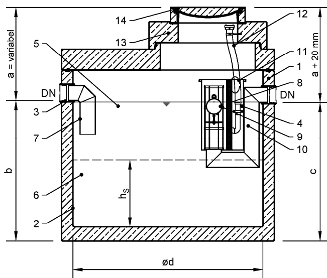
Sedimentations-/ Abscheideeinrichtung NeutraMax
