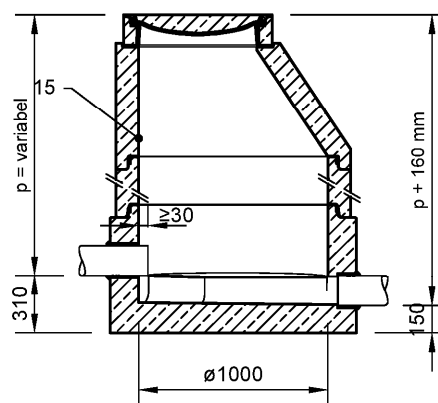
Probenahmeschacht
