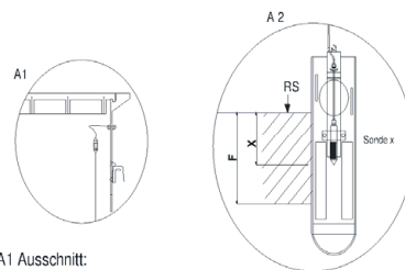
Gefällesprung GF 160 mm Zu- und Ablauf DN 200
