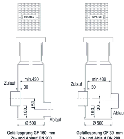
PEHD-Probenahmeschacht
