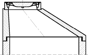
Ausführung mit Schachthals (exzentrisch)
