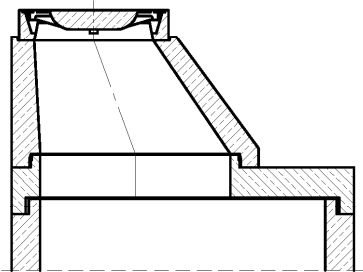
Ausführung mit Übergangsplatte/Schachthals
