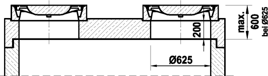
Ausführung mit Abdeckplatte optional mit 2 Wartungsöffnungen
