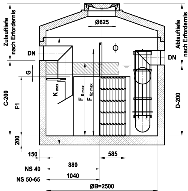
Ausführung mit Schachthals
