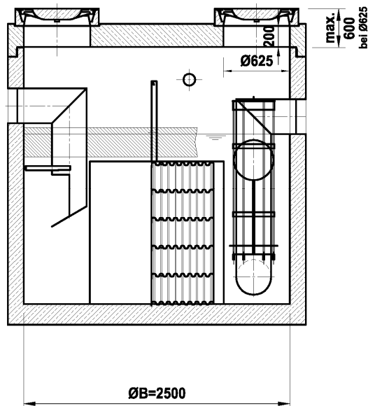
Ausführung mit Abdeckplatte
