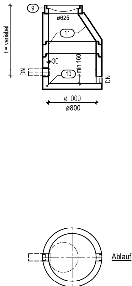
Probenahmeeinrichtung DN 1000/ 800 Ausführung nach DIN 1999-100
