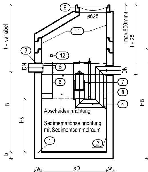
Abscheideeinrichtung Typ Ekotek KA-I System A mit Koaleszenzeinrichtung
