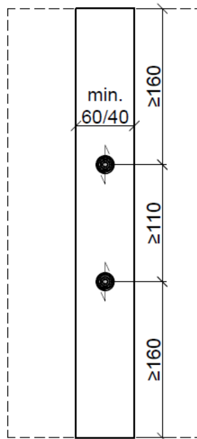
Detail horizontale Verschraubung (Ansicht)
