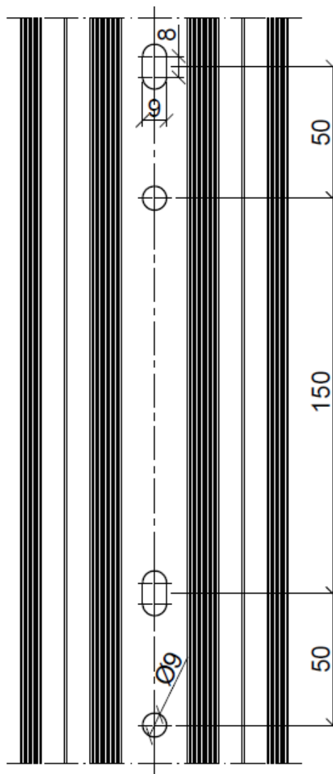
Detail Verschraubung EiSYS-P mit Fassadenprofil 102 x 50 x 2 mm 3 :
