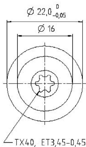
Tellerkopf für Durchmesser 8,0
