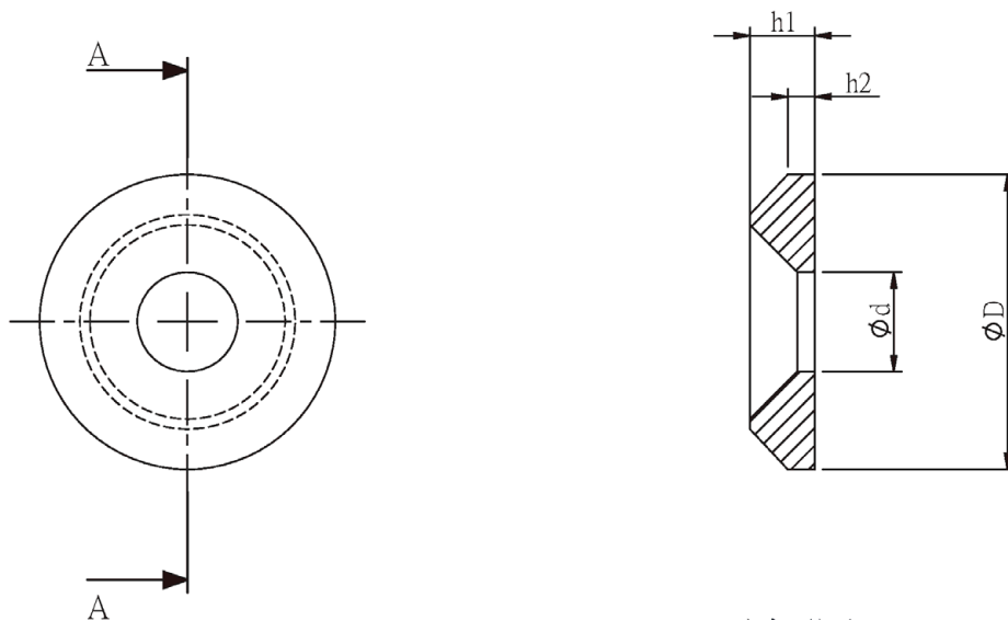
剖面圖 A-A
