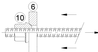
Kugelbundmutter aufgelagert Druck
