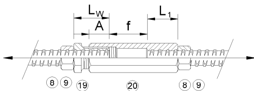
Bild 5 Muffenstoß - Spanschloß Ø12 - 50
