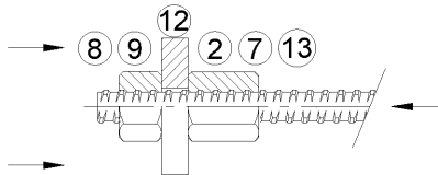
Ankerplatte Druck
