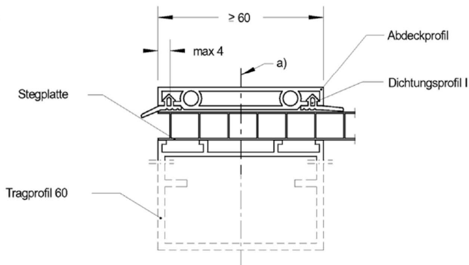
Schnitt A-A
