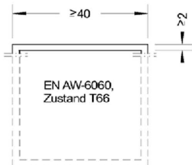
Tragprofil 40
