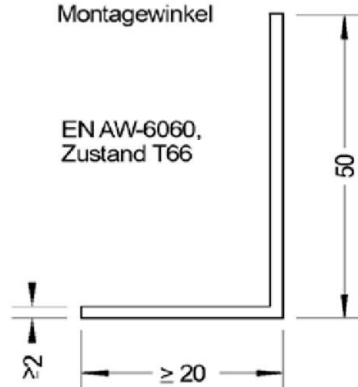
Montagewinkel
