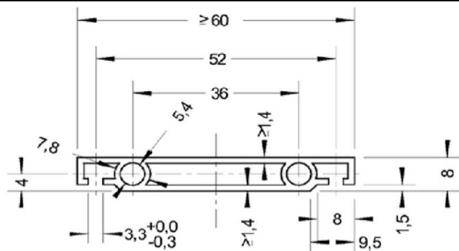
Abdeckprofil
