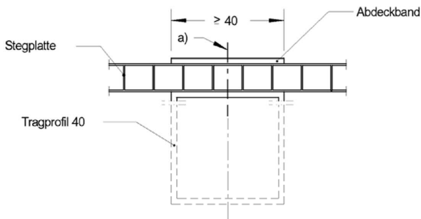
Schnitt C-C
