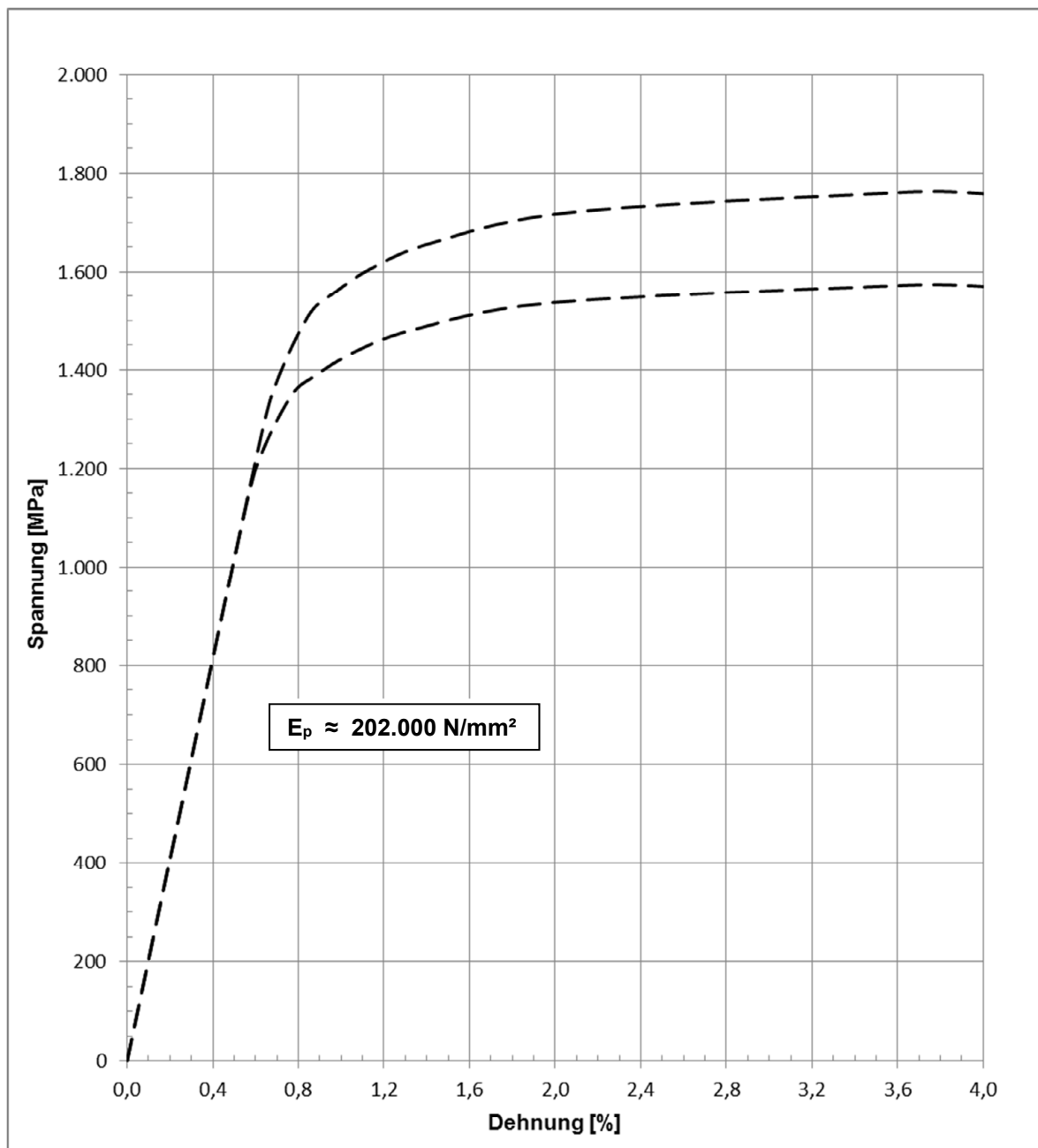
Bild 2: Prinzipieller Spannungs-Dehnungs-Verlauf
