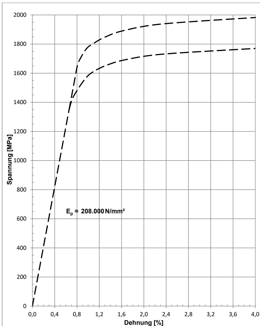
Bild 2: Prinzipieller Spannungs-Dehnungs-Verlauf
