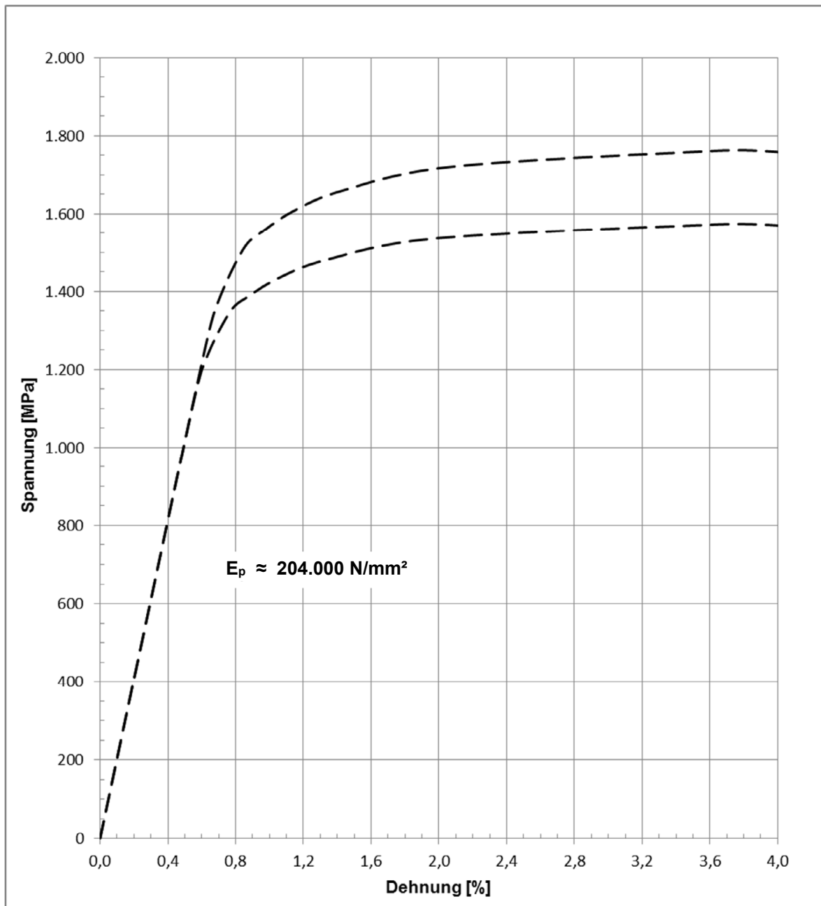
Bild 2: Prinzipieller Spannungs-Dehnungs-Verlauf
