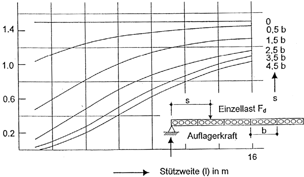
Auflagerkraft am Längsrand infolge Einzellast in Feldmitte
