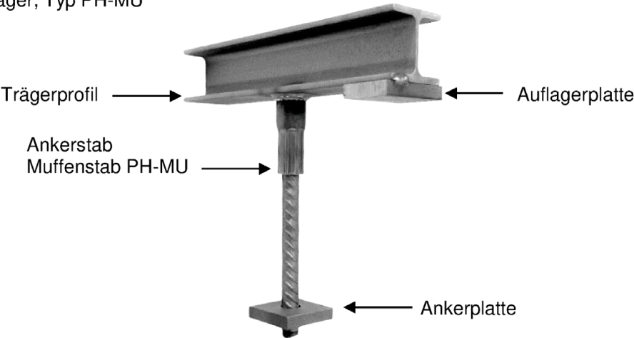
Bild 1.1: PFEIFER-Stahlaufleger, Typ PH-MU
