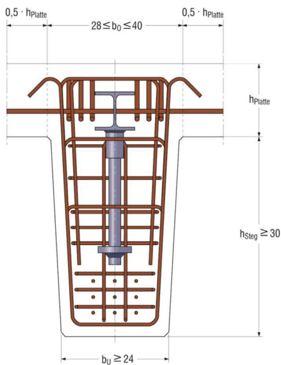
Bild 7: Grundmodul 2
