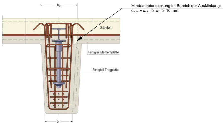
Bild 16: Trogplatte mit Grundmodul
