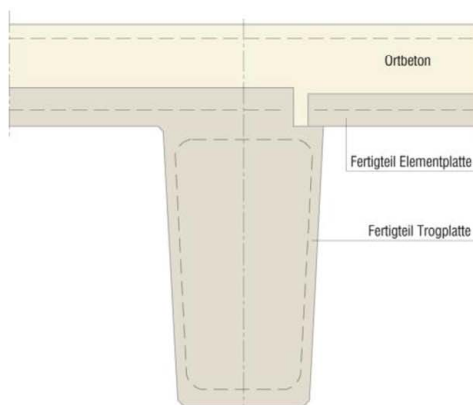
Bild 15: Individueller Querschnitt (Beispiel: Trogplatte mit Elementplatte einseitig)
