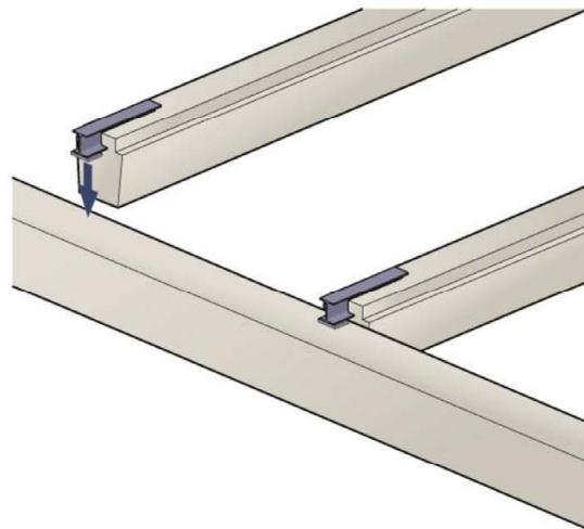
Bild 4: Nebenträger / Unterzüge
