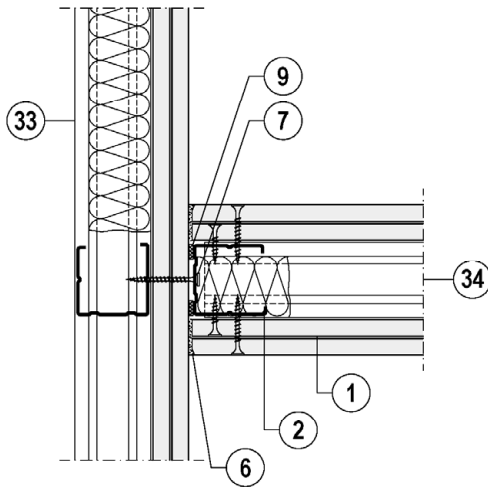
Ausführung bei zu erwartender Wanddurchbiegung \leq 10 mm
