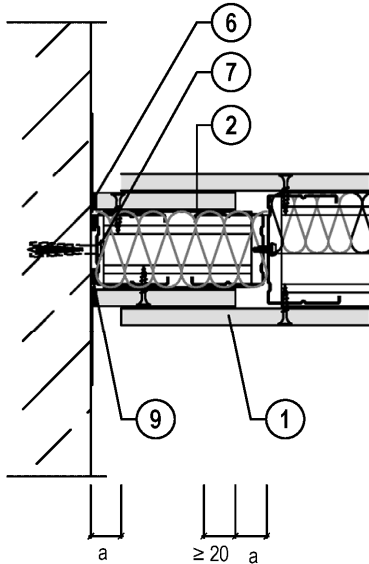
Gleitender Wandanschluss
