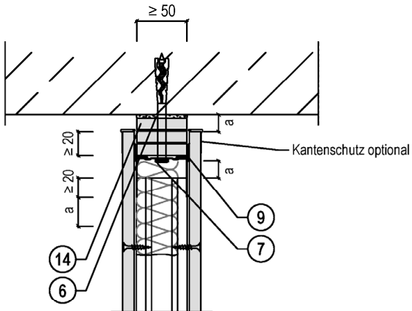
Gleitender Deckenanschluss
