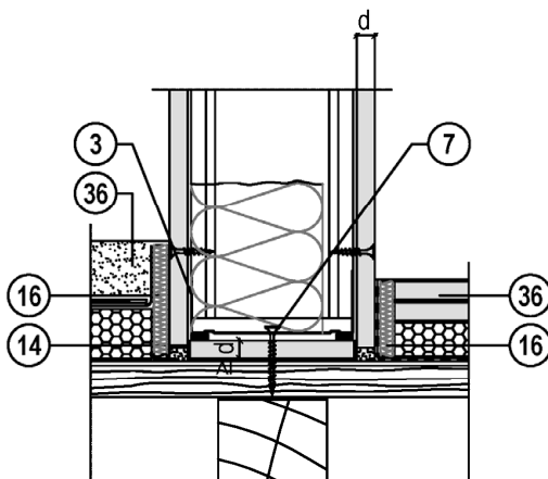
Systemskizze Beispielausführung für Anschlusssituation
