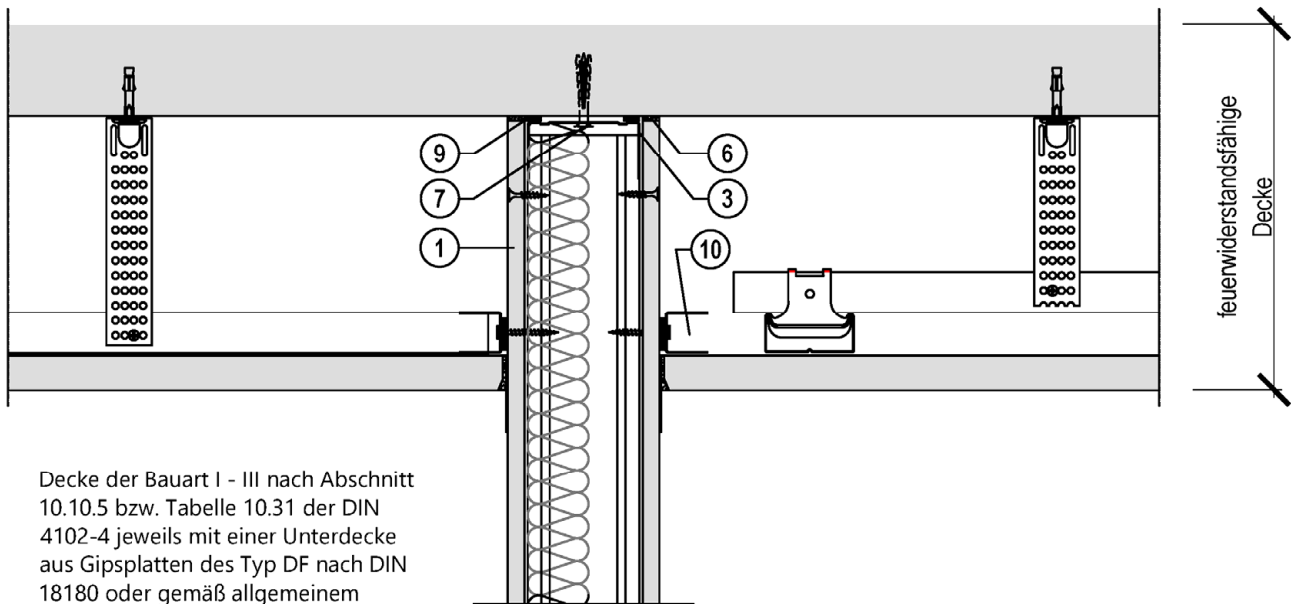
Systemskizze Beispielausführung für Anschlusssituation
