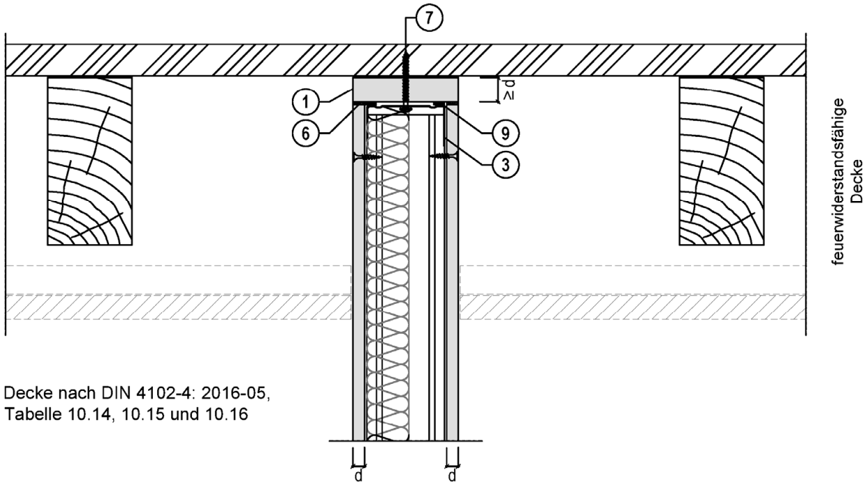
Systemskizze Beispielausführung für Anschlussituation
