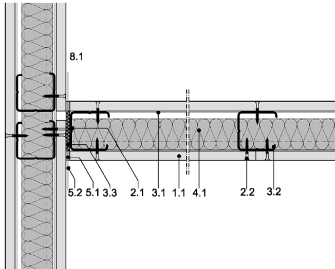
T-Anschluss an eine durchgehende Trennwand mit Trennfuge. Fugenbreite \leq 20\text{mm} Variante 3
