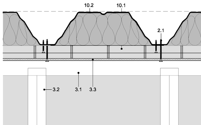
Längsschnitt
