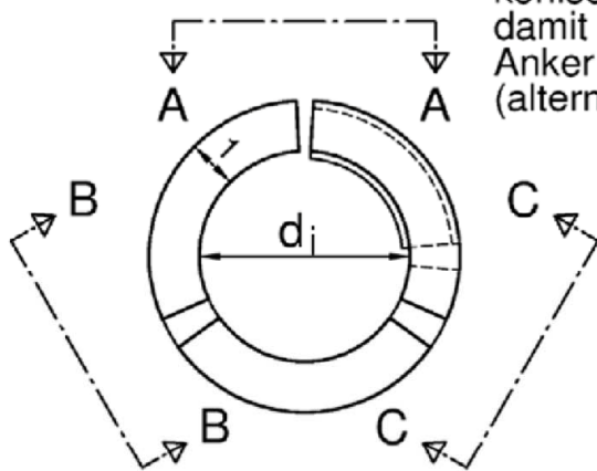
Draufsicht
