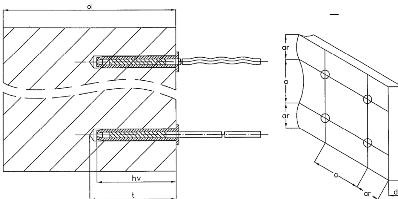
Bauteilabmessung
