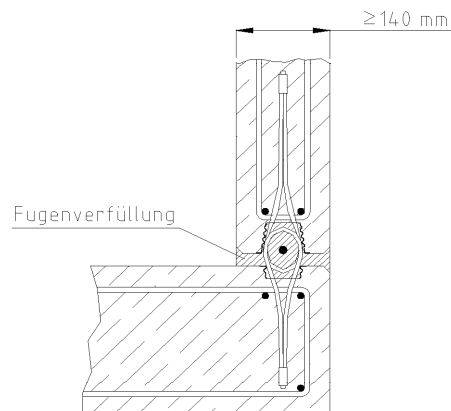
Bild 7: Wand - Wand – Eckverbindung - Regeldetail
