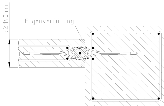
Bild 6: Stützen - Wandverbindung
