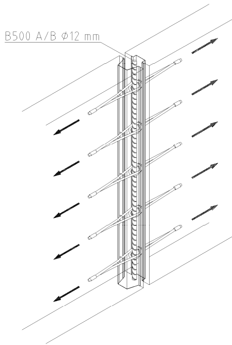
Bild 17: Zugbeanspruchung in Schlaufenlängsrichtung
