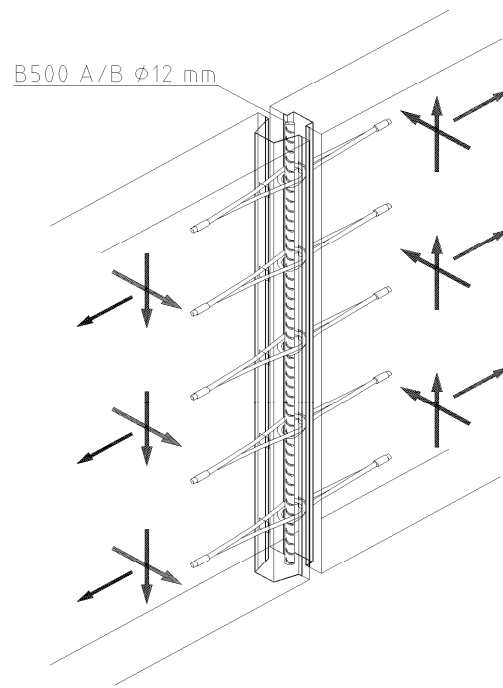
Bild 20: Kombinierte Beanspruchung
