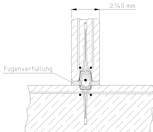
Bild 9: Wand - Wand – T-Verbindung - Regeldetail
