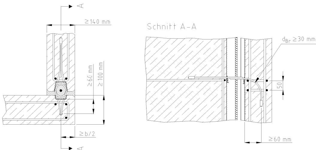
Bild 8: Wand - Wand – Eckverbindung - Detail bei abgewinkelter Seilschleufe
