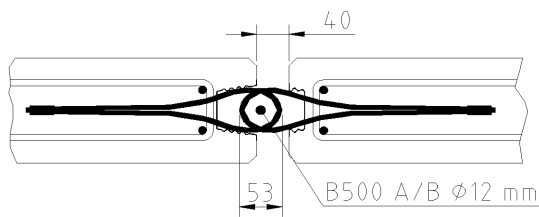
Bild 14: Maximale Fugenbreite
