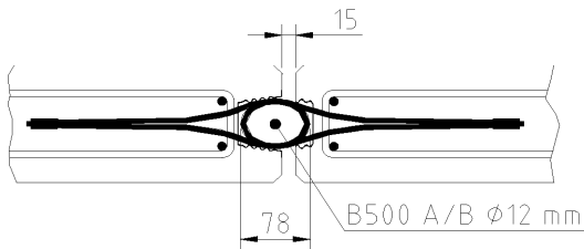
Bild 13: Minimale Fugenbreite
