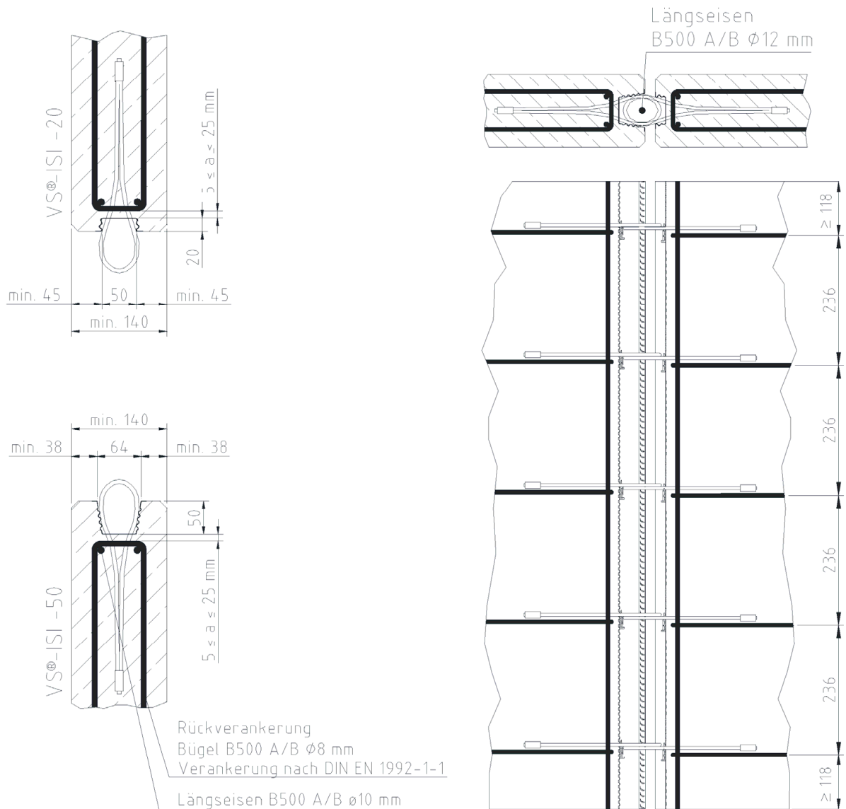
Bild 11: Vergussnut, Bewehrung
