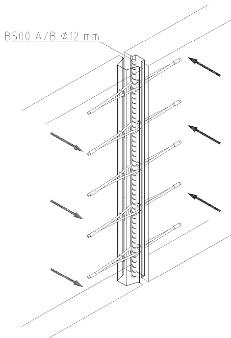
Bild 19: Beanspruchung senkrecht zur Fugenlängsrichtung und Wandebene
