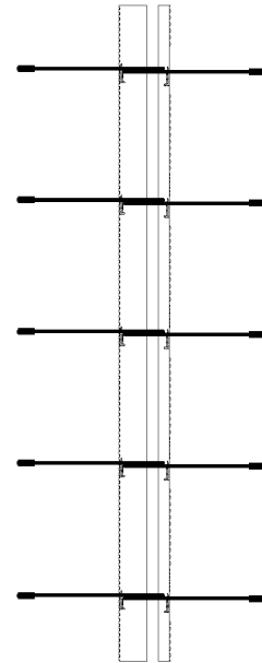
Bild 15: Regeldetail Schlaufenüberlappung
