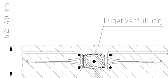
Bild 5: Wand - Wandverbindung
