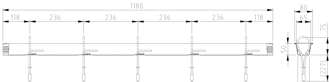
Bild 1: VS®-ISI-50 (Längs- und Querschnitt)
