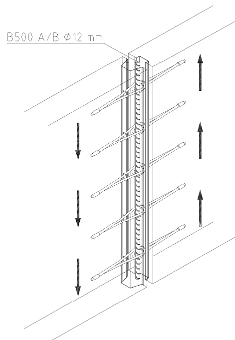
Bild 18: Beanspruchung parallel zur Fugenlängsrichtung
