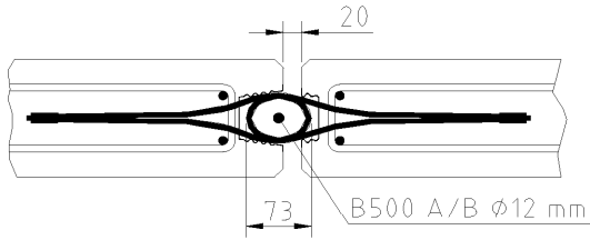
Bild 12: Regeldetail Fuge
