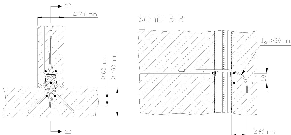
Bild 10: Wand - Wand – T-Verbindung - Detail bei abgewinkelter Seilschleife
